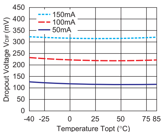
RP103x12xx
