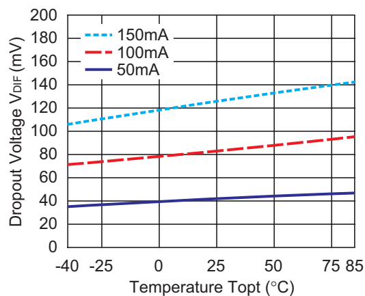
RP103x33xx
