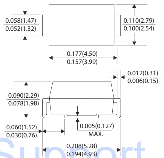
DO-214AC (SMA)
