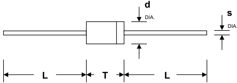
DO-204AC/DO-15
