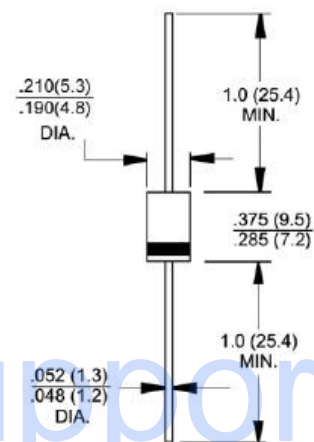
DO-201AD
